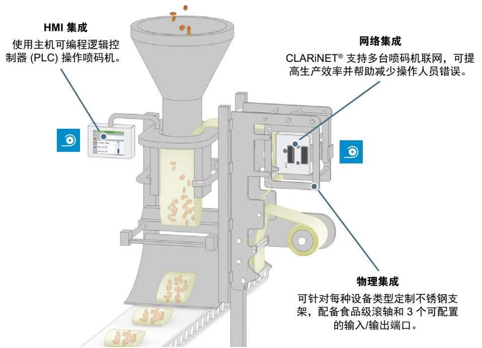
伟迪捷热转印打印 (TTO) 集成到 OEM 制造的肉类和家禽立式充填封口包装机
